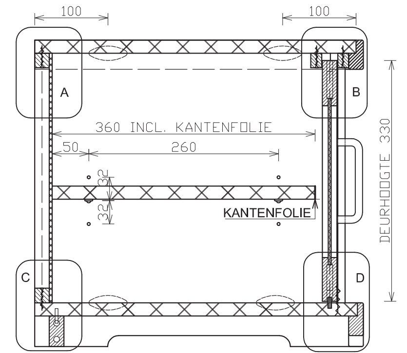
DOORSNEDE A-A
