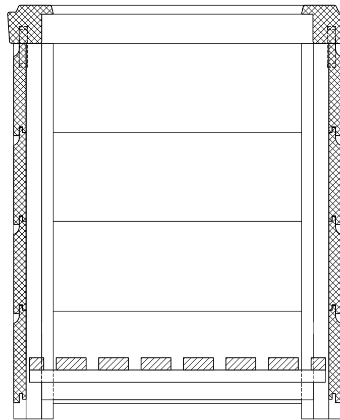
Doorsnede B-B
